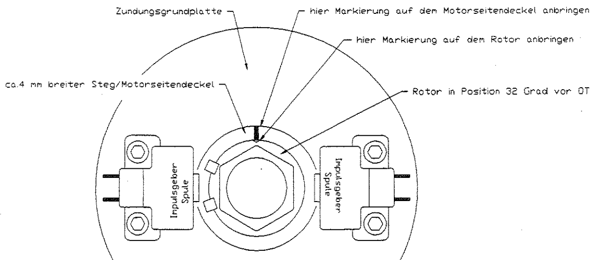
Bild 4.2.2 : Modelle mit Nippon-Denso-Lichtmaschine
