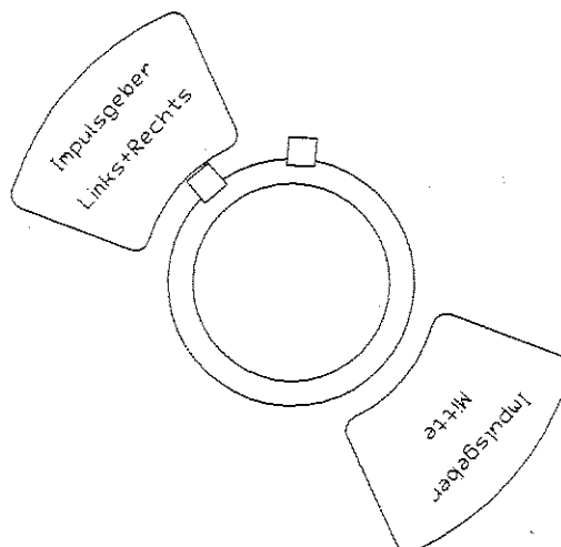
Bild 3.2.1: Montage des Doppelimpulsgebers bei den Modellen mit BOSCH-Lichtmaschine.
