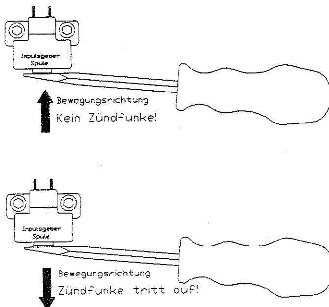
Bild 4.1 : Funktionstest mit dem eingebauten Testprogramm
