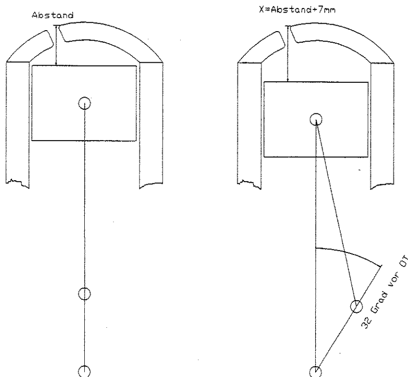
Bild 4.2.1 : Anbringung einer neuen 32 Grad-Markierung
