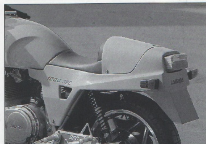
Sitzbankschale SFC Sitzbankpolster Heckbürrzel Rückenkissen
