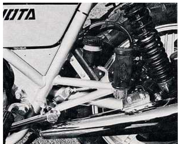
Bild 268 Das Bild zeigt die Einstellschraube des Bremspedals hinter der Fußrasten
