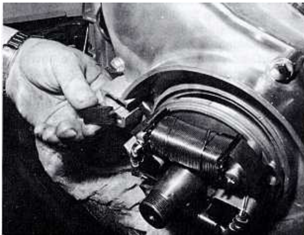
Bild 198 Dieser Gummistopfen muss in der richtigen Orientierung eingesetzt werden, sonst scheuert er nach dem Aufsetzen des Schwungrades das Kabel durch
