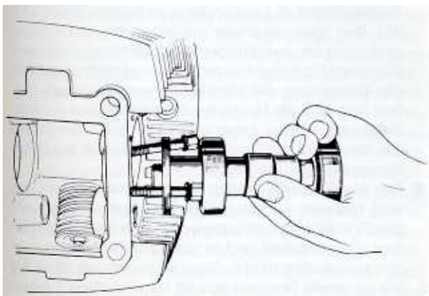
Bild 87 Mit den beiden Schrauben wird die Nockenwellenhälfte am Kettenrad befestigt
