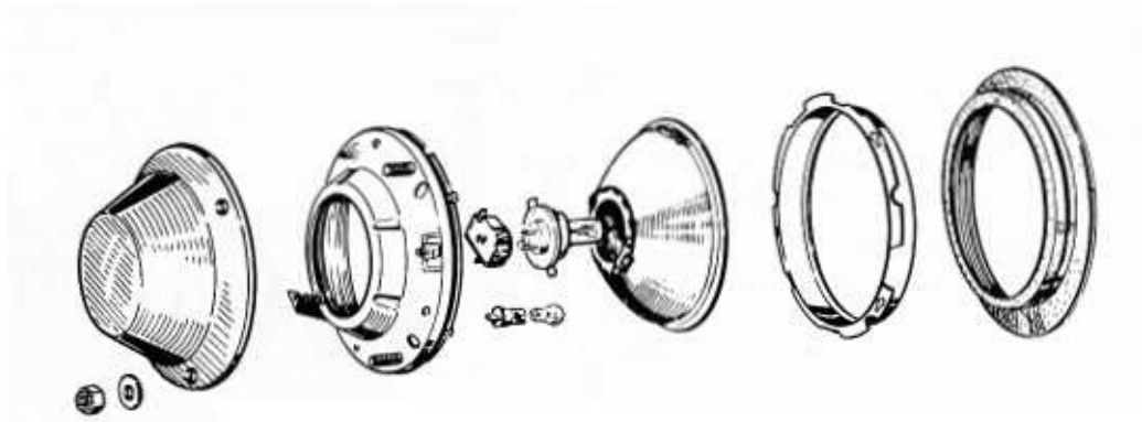
Bild 185 Der Carello-Scheinwerfer der SFC (1975 und in anderen Jahren eingebaut)
