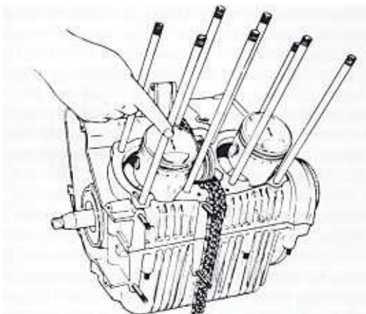
Bild 111 An allen Modellen muss der Pfeil auf dem Kolbenboden nach vorn zeigen
