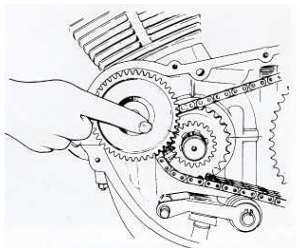
Bild 125 Der Finger zeigt auf die beiden Marken an den Zahnradern
