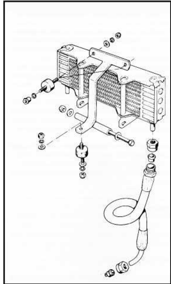
Bild 130 Der Ölkühler der neueren Dreizylinder. Die älteren Dreizylinder und die SFC benutzen ähnliche Kühler
