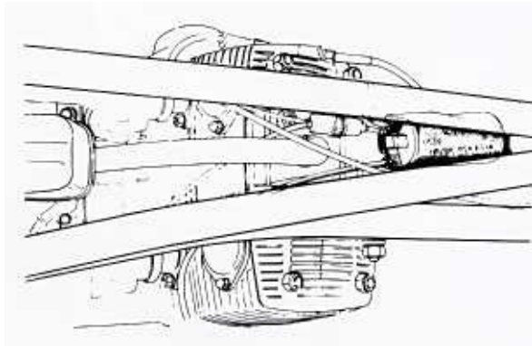
Bild 219 Die Zündspule der SFC
