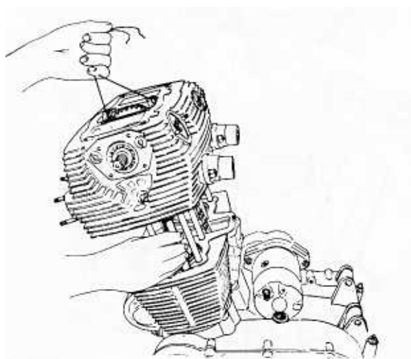
Bild 108 Beim Absenken des Zylinderkopfes werden die Steuerkettenenden durch den Kettenschacht gezogen
