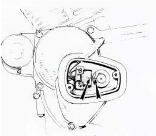
Bild 217 Mit der Kurbelwelle im oberen Totpunkt (d.h. die Kurbelwellenmarke an der anderen Motorseite fluchtet mit der Gehäusemarke) müssen die beiden mit Pfeilen bezeichneten Marken fluchten (SFC mit BTZ)
