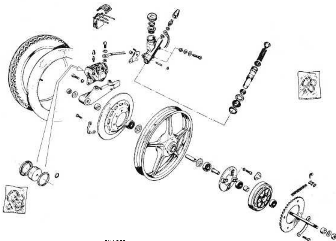
Bild 252 Die hintere Scheibenbremse an Gussrädern
