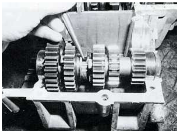
Bild 151 Diese Schaltklauen dürfen nicht abgenutzt oder abgerundet sein
