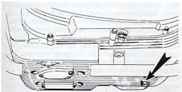
Bild 40 Der Pfeil zeigt auf die Ölabblassschraube der Dreizylinder
