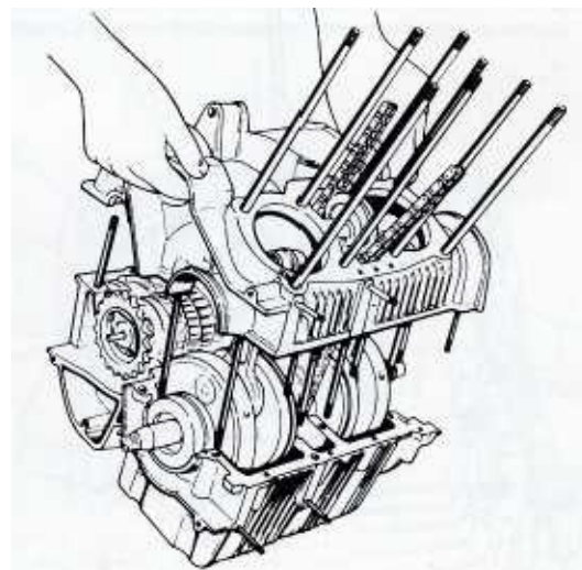
Bild 88 An dieser Stelle müssen die Enden der Steuerkette mit Draht gesichert werden
