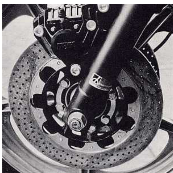
Bild 272 Die gelochte Bremsscheibe der Jubiläums-1200er. Ebenfalls sichtbar sind die Sicherungsbleche der Befestigungsschrauben der Bremsscheibe an der Radnabe
