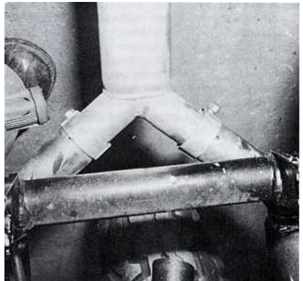
Bild 178 Der hintere Teil des Sammelrohres der Auspuffanlage am Dreizylinder (drei-in-eins- in -zwei); das Teil stammt von Laverda selbst
