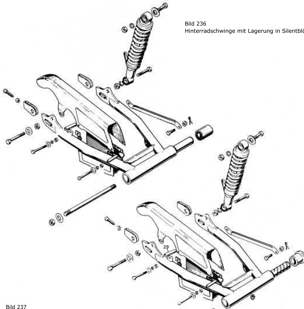
Bild 237 Hinterradschwinge mit Lagerung in Bronzebüchsen; in der Mitte des Querrohrs der Schmiernippel
