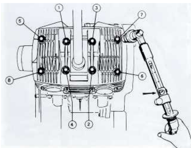
Bild 93 Anzugsreihenfolge der Zylinderkopfschrauben am Zweizylinder
