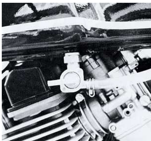
Bild 54 Ein Kraftstoffhahn neuester Ausführung aus Kunststoff. Zum Zerlegen nimmt man den mit zwei Schrauben befestigten Flansch ab. Es handelt sich hier um eine Jubiläums -1200er
