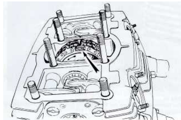
Bild 92 Das offene Ende der Schliessfeder muss nach hinten zeigen
