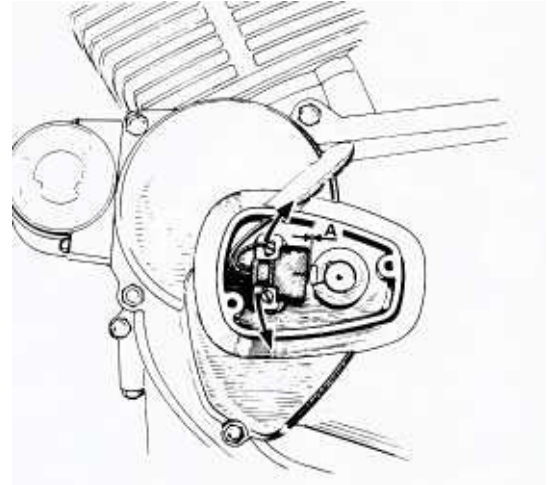
Bild 218 Messen des Spiels (A) zwischen Impulsgebernocken und Impuls-aufnehmer an der SFC mit BTZ
