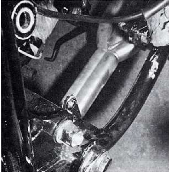
Bild 78 Die Motorbefestigung eines Dreizylinders am Rahmen bei ausgebautem Motor. Der Lappen zum Schutz des vorderen Rahmenrohrs war zu kurz, deshalb die abgeplatzte Farbe
