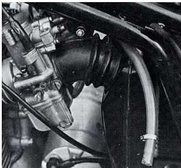
Bild 51 Ein Luftfilter der zweiten Generation an einer SF. Der Filter ist nicht leicht auszubauen, da er fest sitzt
