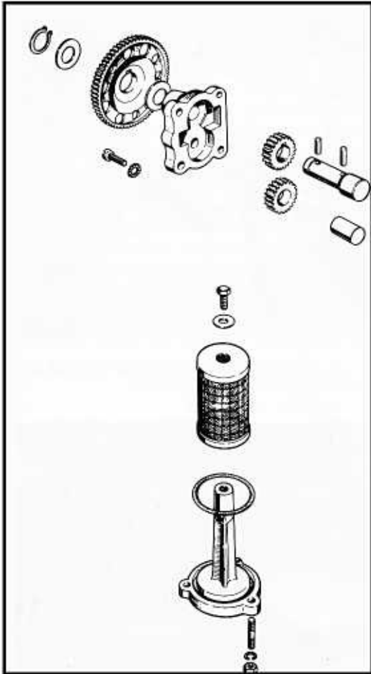
Bild 129 Ölpumpe und Ölfilter des Dreizylinder
