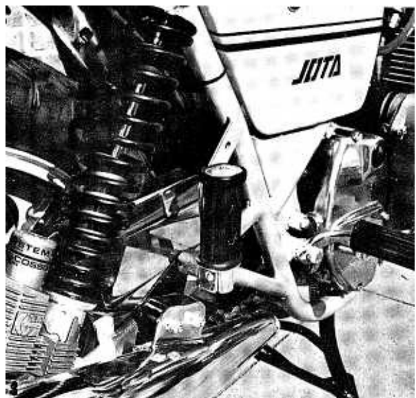
Bild 235 Eine 79er Jota mit Federbeinen von Corte e Cosso
