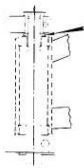
Bild 233 Querschnitt durch den Lenkkopf; der Pfeil zeigt auf die Einstellmutter
