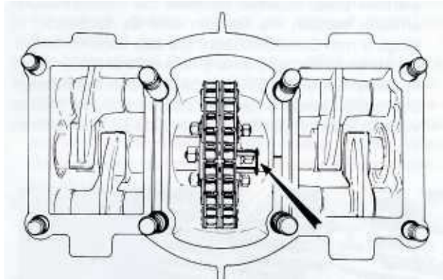
Bild 91 Das Kettenschloss muss so eingesetzt werden, wie die Abbildung zeigt
