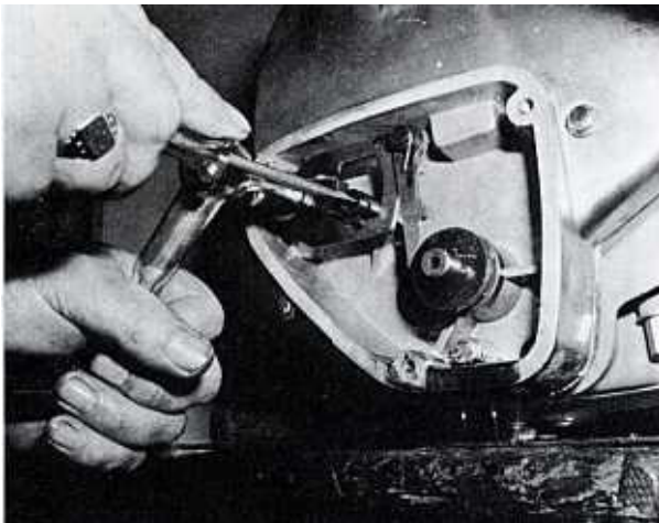
Bild 144 Einstellen der Exzentrerschraube für gleichen Schalthebelweg nach oben und unten
