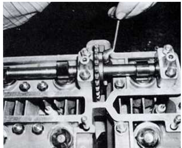
Bild 68 Die eingebaute Nockenwelle soll noch vor dem Anziehen der Lager so gedreht werden, dass kein Ventil geöffnet ist
