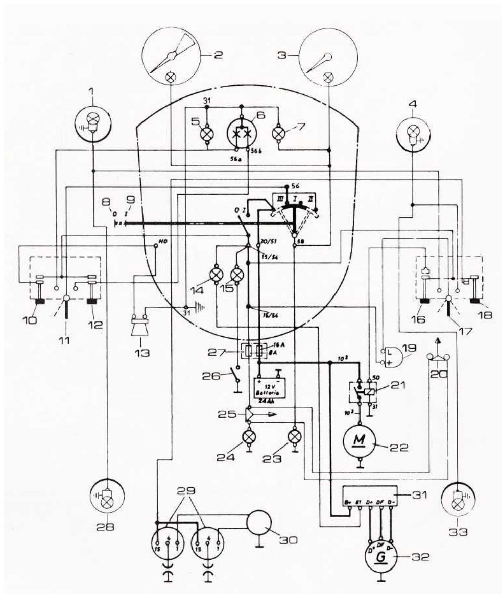
Bild 275 Schaltplan 750GT 1972/74 mit »langem« Bosch-Scheinwerfer, Schmith-Instrumenten und Lucas-Schaltern
