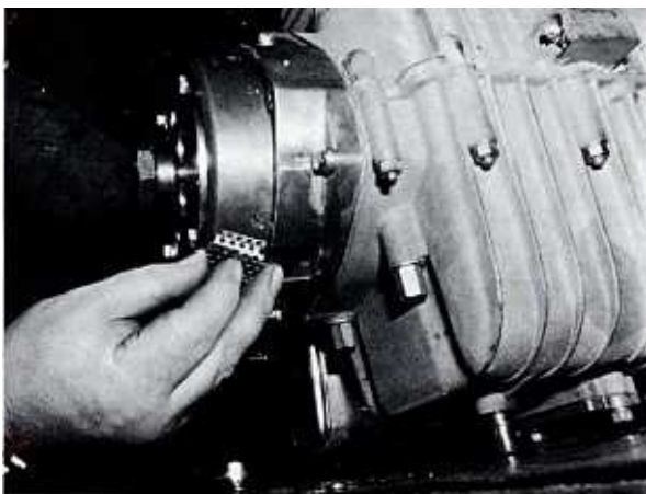
Bild 196 Das Schutzgitter der Lüftungsöffnung an der Lichtmaschine des Dreizylinders muss immer eingesetzt sein, sonst können Steine eindringen
