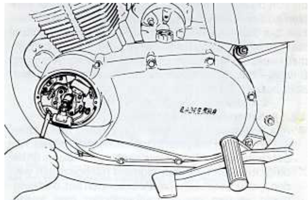
Bild 46 Einstellen des Zündzeitpunktes. Der Schraubendreher ist an einer der drei Befestigungsschrauben der Unterbrechergrundplatte angesetzt (Zweizylinder)
