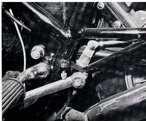
Bild 267 Die Standardausführung (links) des Bremspedals für die Scheibenbremse
