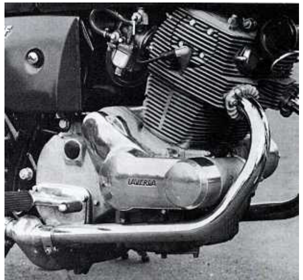
Bild 176 Die spätere Auspuffanlage des Zweizylindermotors mit der grossen Ausgleichskammer unter dem Getriebe; diese wird mit einer grossen Schelle befestigt, die bald zum Rosten neigt
