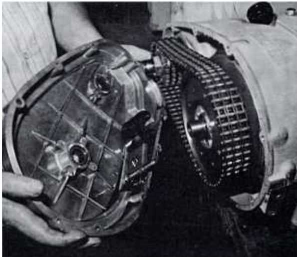
Bild 113 Ausbau des Primärtriebsdeckels an einem neueren Dreizylinder, erkennbar am Kettenspanner
