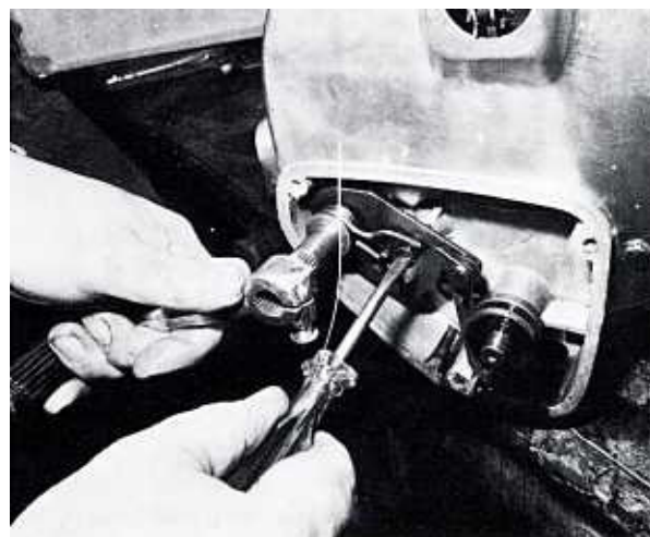
Bild 143 Der Schraubendreher ist am Exzenter angesetzt
