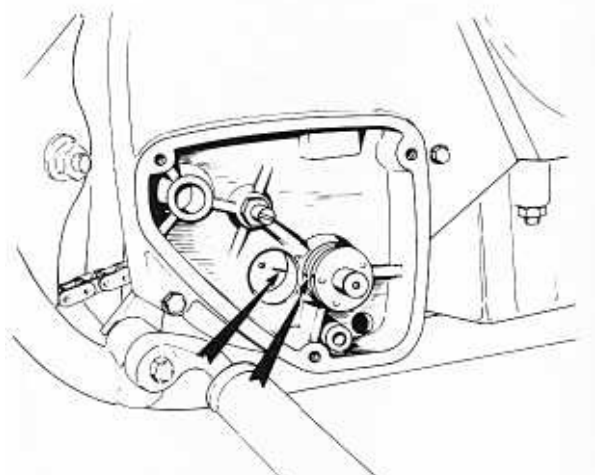
Bild 145 Die beiden Pfeile zeigen auf die Einstellmarken der Schalwelle und der Schaltwalzenwelle
