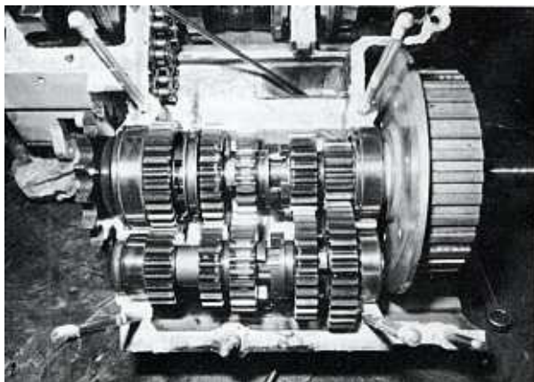
Bild 150 Die Getriebewellen mit der Kupplungs rechts und dem Getrieberitzel links
