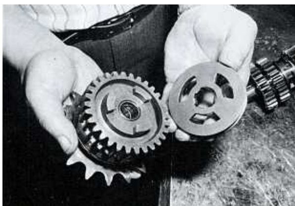
Bild 152 Die Schiebemuffe muss gegenüber den Schaltklauen des 5. Ganges auf der Hauptwelle liegen, wie das Bild zeigt
