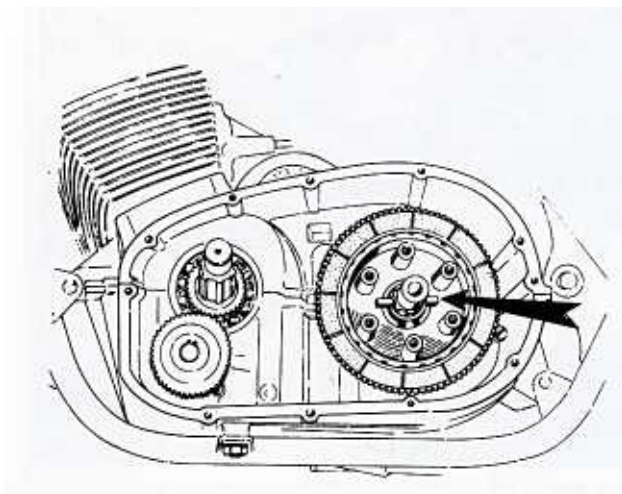
Bild 124 Der Pfeil zeigt auf den Befestigungsstift der Kupplungsgrundplatte
