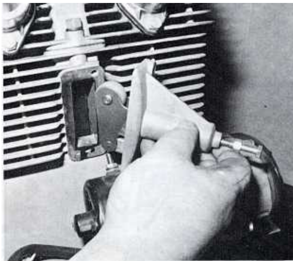
Bild 94 Die Gewindebohrungen zur Befestigung des Steuerkettenspanners liegen aussermittig
