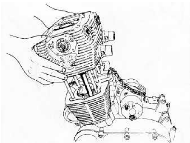
Bild 107 Der Zylinderkopf wird zuerst auf einer Holzunterlage auf den Stiftschrauben abgestellt
