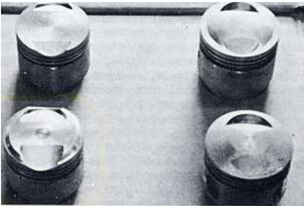
Bild 109 Die linken Kolben gehören zur 1000er Dreizylinder, der obere zur 3CL, der untere mit höherer Verdichtung gehört zu einer Jota. Rechts 750er Kolben, oben zu einer SF, unten zu einer SFC mit hoher Verdichtung
