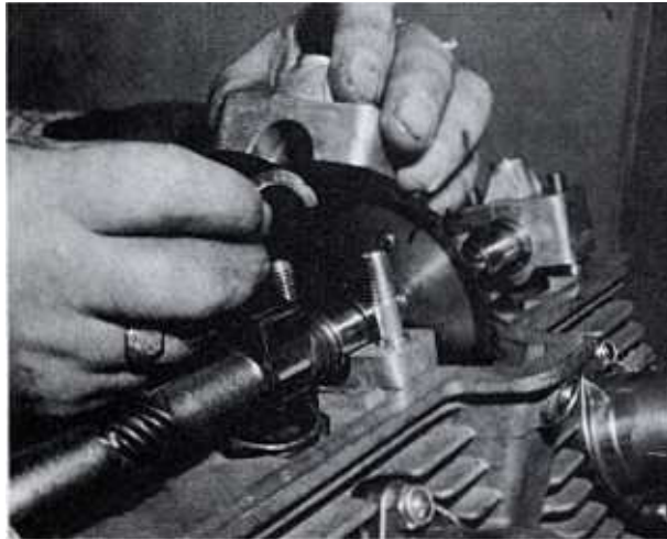
Bild 67 Beim Zusammenbau dürfen die Einstellscheiben der Nockenwellenlager nicht vergessen werden
