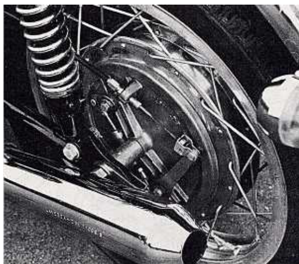
Bild 261 Die neuere Laverda-Trommelbremse ist baugleich mit der Vorderradbremse.
