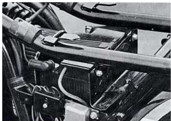
Bild 36 Die Unterbringung der Batterie an den späteren Zweizylindermaschinen. Man beachte das Gummiband über der Batterie und den engen Zwischenraum zwischen Batterie und Rahmen
