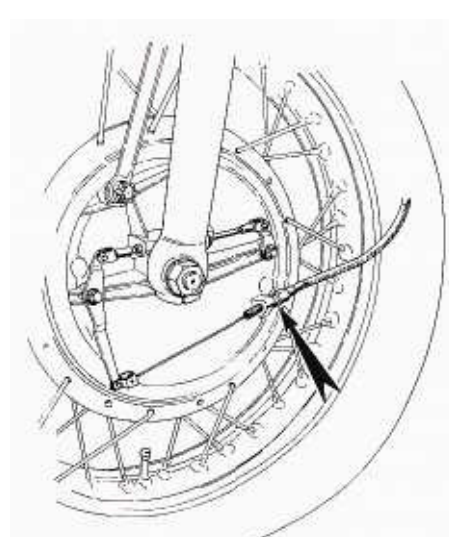
Bild 256 Die Einstellschraube für den Bremszug an der Laverda-Bremse
