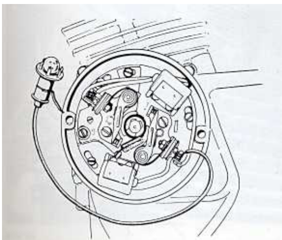
Bild 47 Anschliessen einer Kontrollampe zum Einstellen des Zündzeitpunktes
