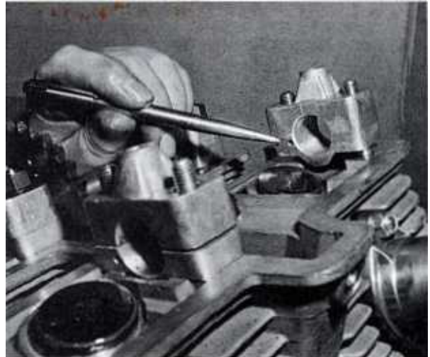
Bild 66 Der Stift zeigt auf die Ölbohrung des Nockenwellenlagers. Bei verkehrtem Einbau läuft die Nockenwelle trocken, aber nicht lange!
