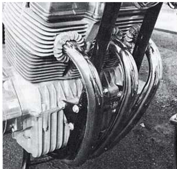
Bild 177 Dieses Bild eines älteren Dreizylinders zeigt die ausgesprochen saubere Führung. Die Auspuffrohre dürfen die Rahmenrohre nicht berühren
