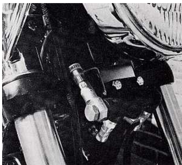
Bild 265 An einigen Dreizylindern ist das Verteilerstück nicht direkt, sondern zeigt ebenfalls den Gummipuffer der Scheinwerferbefestigung
