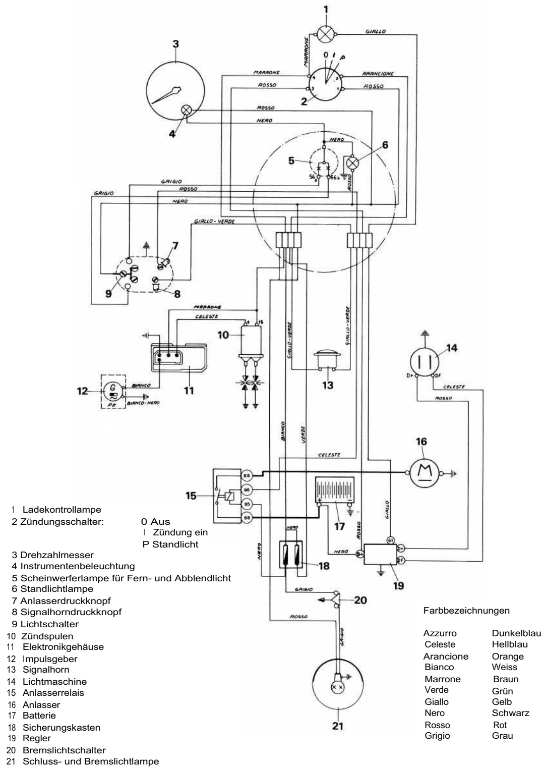
Bild 279 Schaltplan zur SFC mit BTZ um etwa 1975
