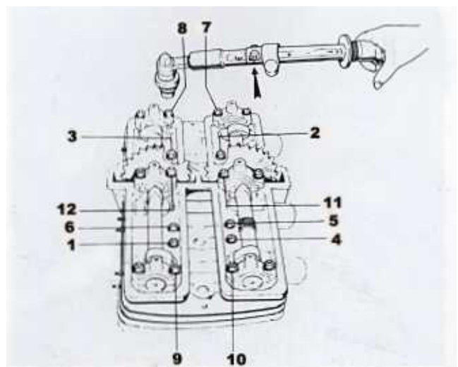
Bild 70 Anzugsreihenfolge der Zylinderkopfschrauben des Dreizylinders
