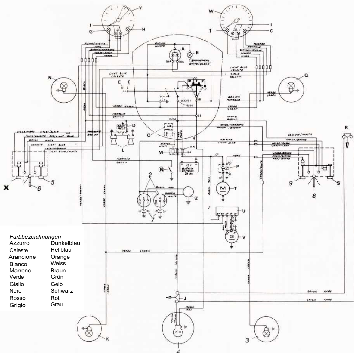
Bild 276 Schaltplan zu 750SF 1972 mit Bosch-Scheinwerfer, Nippon Denso-Instrumenten und Lucas-Schaltern. Maschinen mit dieser Ausrüstung sind selten; die meisten haben zum Bosch-Scheinwerfer auch Bosch-Schalter
