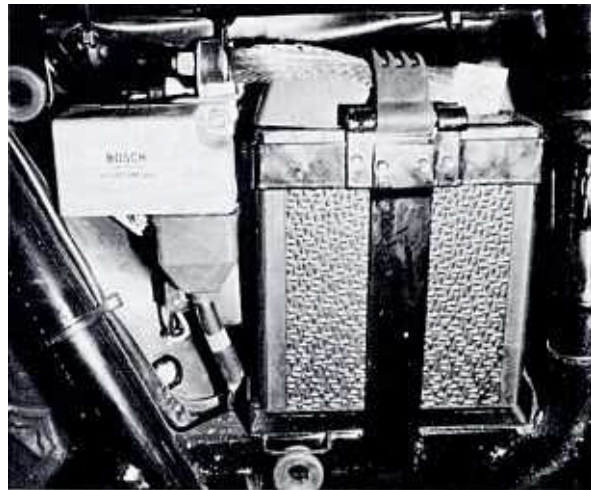
Bild 214 Hinter dem rechten Seitenteil einer mit BTZ ausgerüsteten Maschine findet man eines der so teuren Elektronikkästchen, die aber sehr zuverlässig arbeiten
