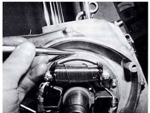
Bild 199 Beim Einbau der Grundplatte müssen die beiden gezeigten Marken aufeinander ausgerichtet werden
