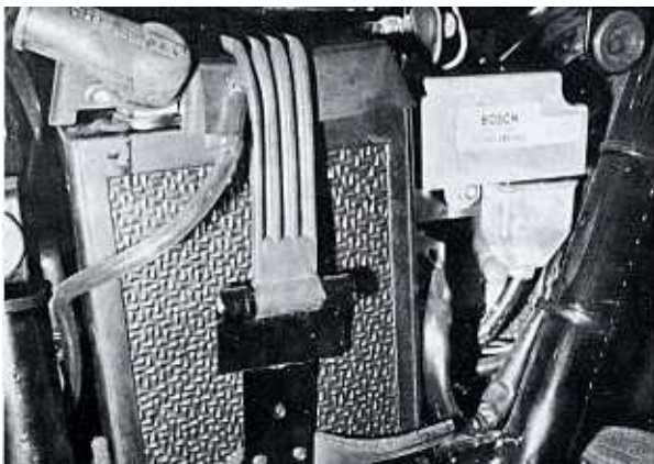
Bild 37 Batteriehalter und -befestigung an einer Dreizylinder, in diesem Fall an einer Maschine mit Hochspannungs-Kondensatorzündung
