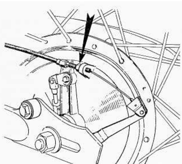
Bild 258 Die Einstellschraube der hinteren Grimeca-Trommelbremse
