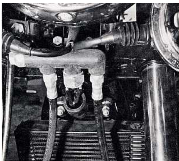
Bild 264 Der Verteiler für die Bremsleitungen an der unteren Gabelbrücke mit abgezogener Kappe über dem Bremslichtschalter
