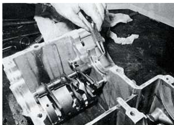
Bild 153 Einsetzen des Sicherungsstiftes der Schaltgabelachse
