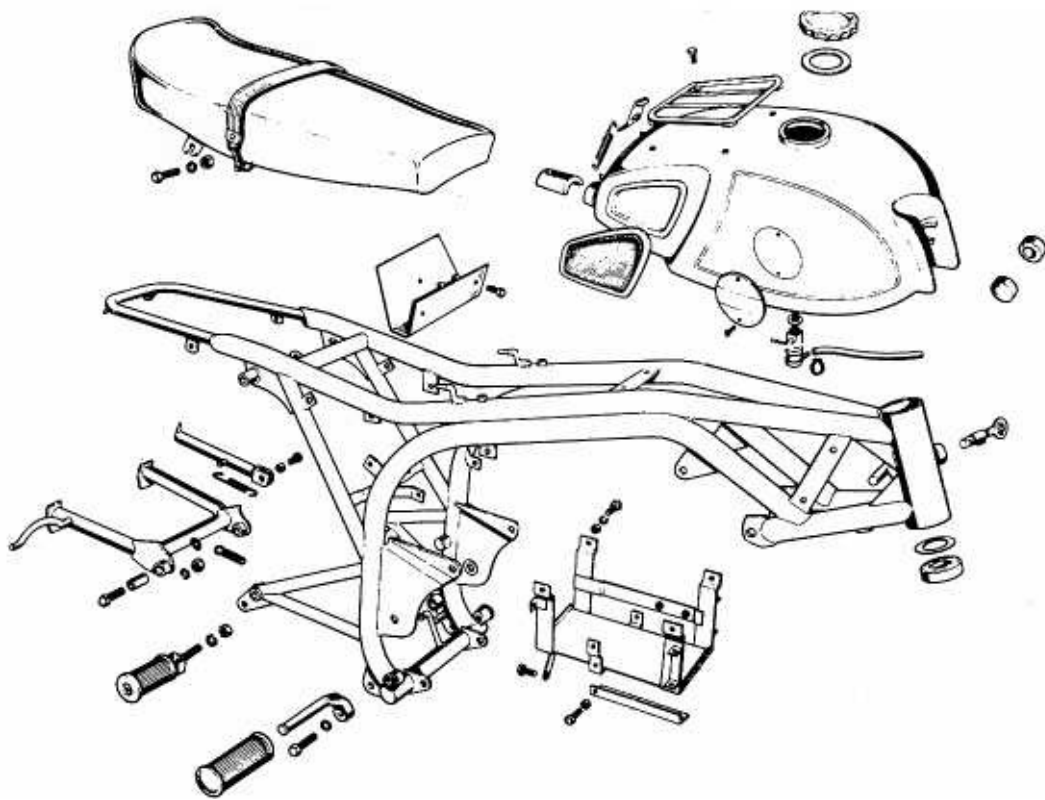
Bild 227 Die älterer Rahmen der 750 GT mit Kraftstofftank
