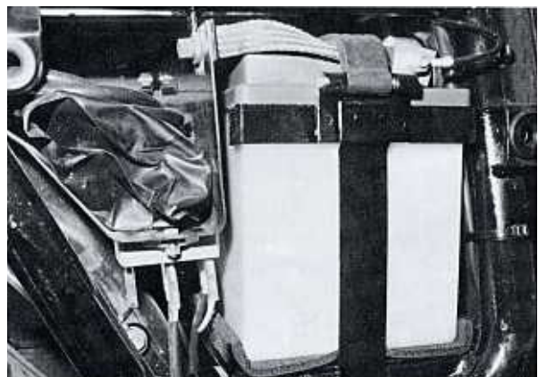
Bild 38 Batteriehalter einer jüngeren Dreizylinder mit Batterie-Transistorzündung mit Kunststoffgehäuse und Metallhaltebügel
