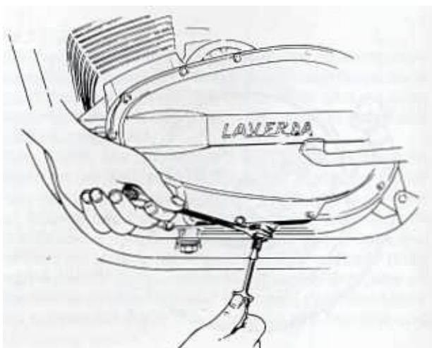
Bild 50 Einstellen des Primärkettenspanners an einem Dreizylinder. Das Bild gilt auch für die Zweizylinder
