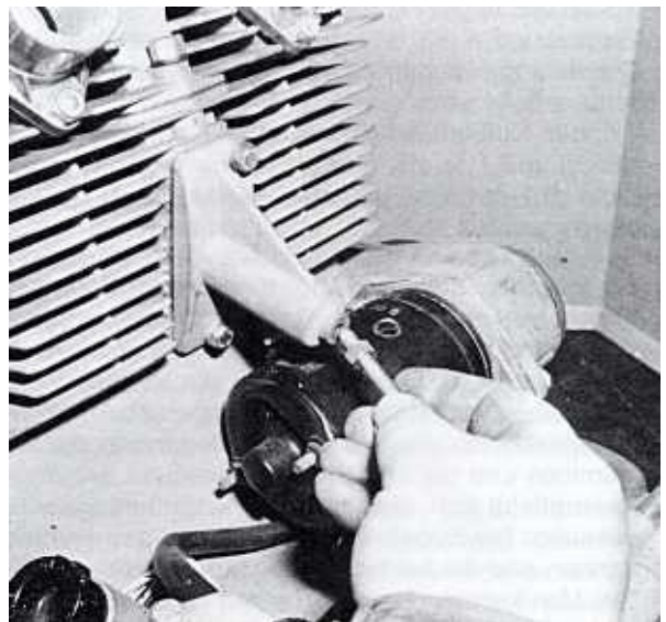
Bild 80 Es empfiehlt sich, vor dem Ausbau des Kettenspanners die Einstellschraube herauszudrehen
