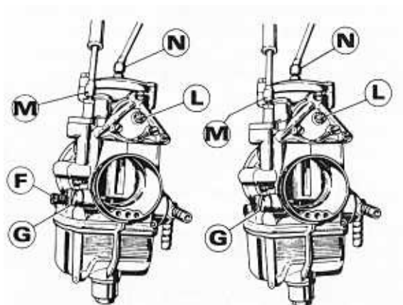
Bild 171 Blick in die Ansaugkanäle der beiden PHF-Vergaser
