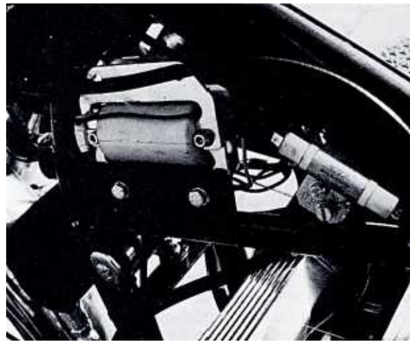
Bild 212 Die andere Zündspule der BTZ. Der weisse Zylinder rechts der Zündspule ist ein Widerstand
