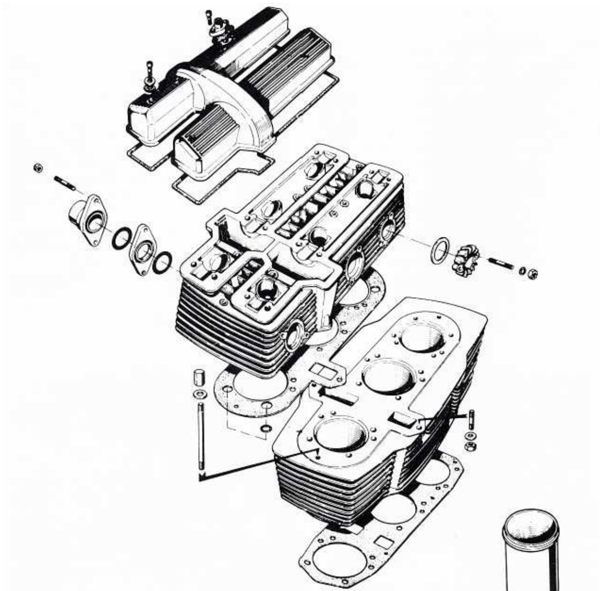
Bild 101 Zylinderkopf und Zylinderblock des Dreizylinders
