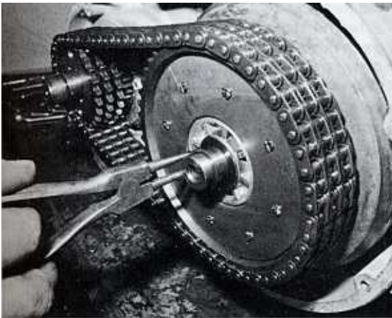
Bild 120 Die Kurbelwellenmutter ist bereits abgeschraubt, der Sicherungsring der Kupplungswelle wird entfernt
