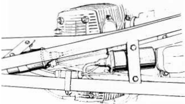
Bild 204 Die beiden Zündspulen des Zweizylinders von oben
