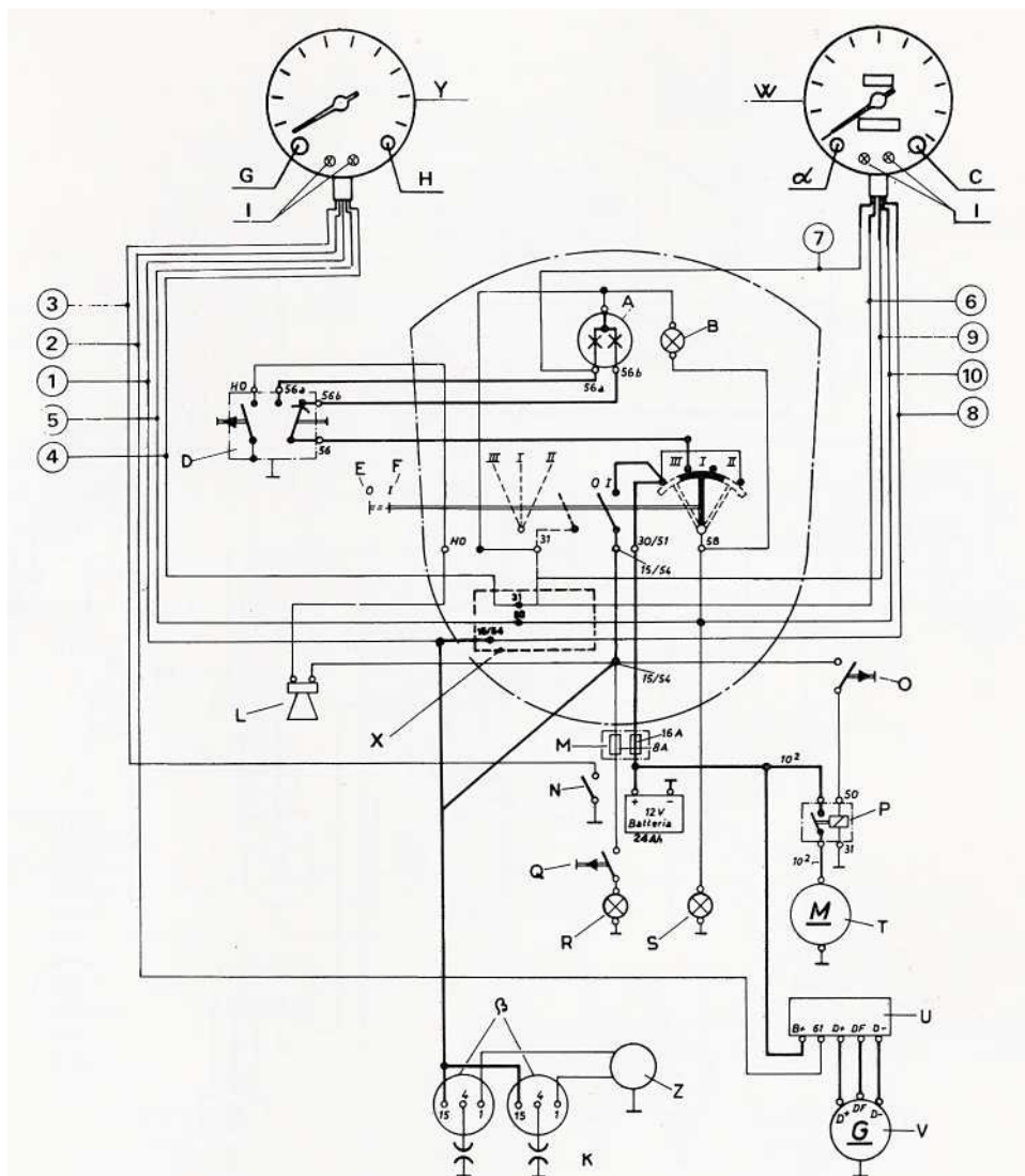
Bild 274 Schaltplan 750SF 1970/71
