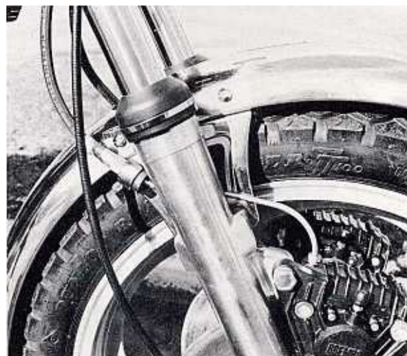
Bild 262 Die Führung der Bremsleitung an einer Dreizylinder mit Marzocchi - Gabel. Alle anderen Maschinen mit Scheibenbremsen sind ähnlich gebaut. Links vom Gleitrohr eine Gummiteile zur Führung der Bremsleitung.
