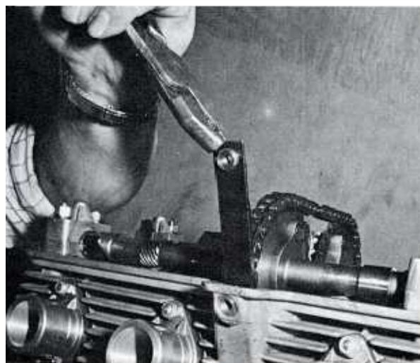
Bild 99 Herausziehen der Gleitschiene des Kettenspanners mit einer Zange
