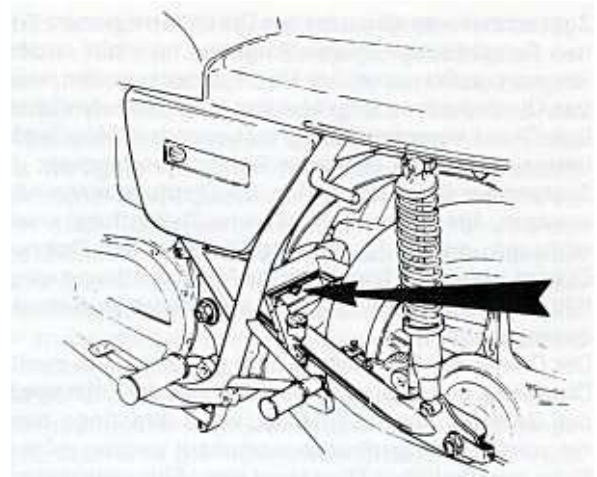
Bild 42 Der Schmiernippel des Schwingenlagers (nur an Lagern mit Bronzebüchsen oder Nadellagern) ist von der Unterseite her zugänglich
