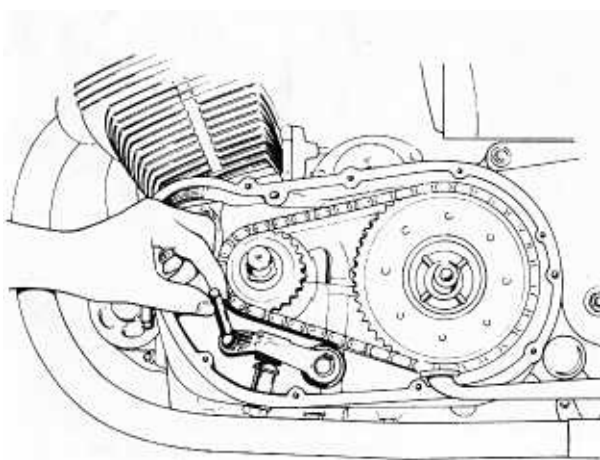
Bild 116 Der Lagerzapfen des Kettenspanners am Zweizylinder
