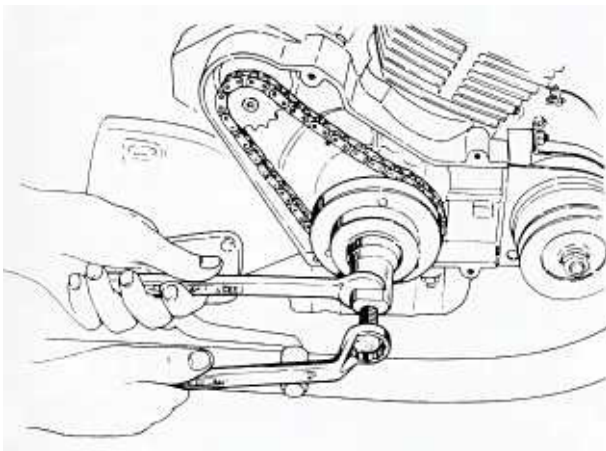
Bild 202 Abziehen des Anlasserfreilaufs mit Spezialwerkzeug am Zweizylinder
