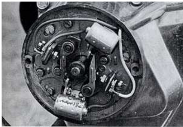
Bild 45 Der Unterbrecher der Zweizylinder
