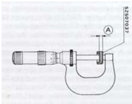
Bild 65 Messen der Dicke der Ventileinstellscheibe für den Dreizylinder
