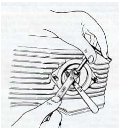
Bild 49 Das Einstellen des Ventilspiels am Zweizylinder ist nicht ganz so einfach, wie man aus dem Bild vermuten könnte
