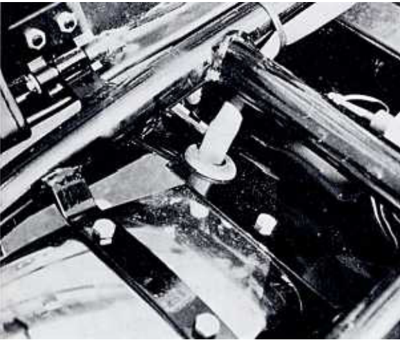
Bild 213 Dieses gelbe Kabel, das durch den hinteren Kotflügel führt, ist nur an Maschinen mit BTZ vorhanden
