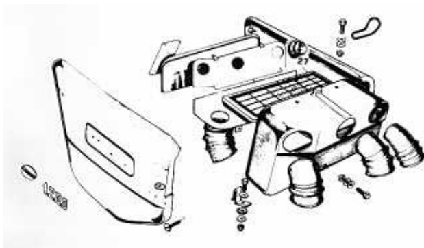
Bild 161 Der Luftfilter der Dreizylinder unterscheidet sich stark von jenem der Zweizylinder
