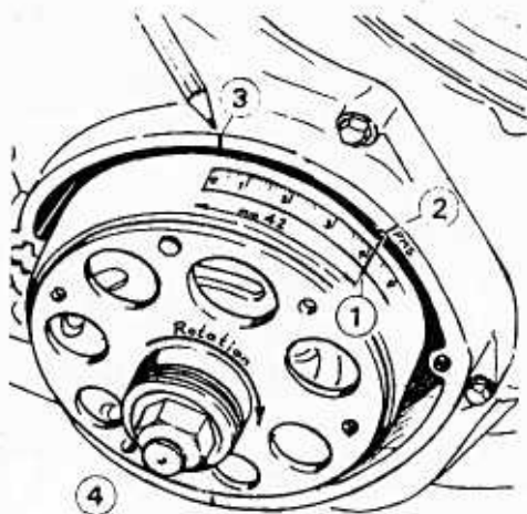
Bild 208 Laverdas Methode zum Prüfen des Zündzeitpunktes an einer Dreizylinder mit BTZ. Die Bedeutung der Zahlen ist die gleiche wie in Bild 207
