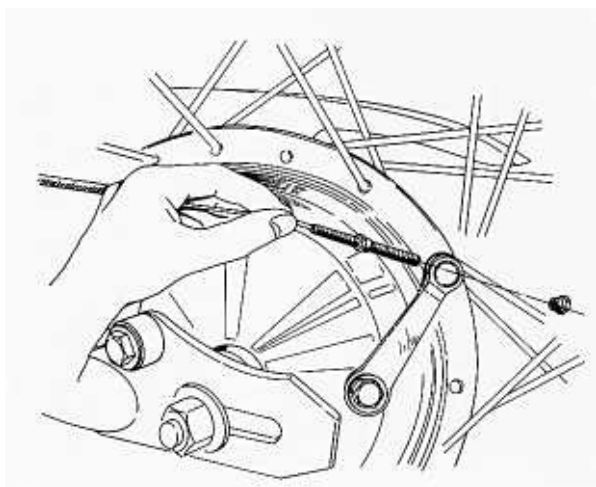
Bild 259 Die ältere Befestigung des Bremsseils an der Laverda-Bremse mit Hilfe der Einstellschraube
