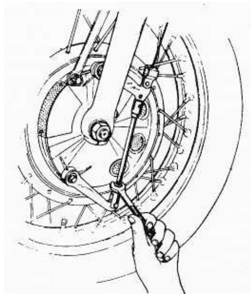
Bild 254 Einstellen der Verbindungsstange zwischen beiden Bremsnockenhebeln an der Grimeca-Bremse
