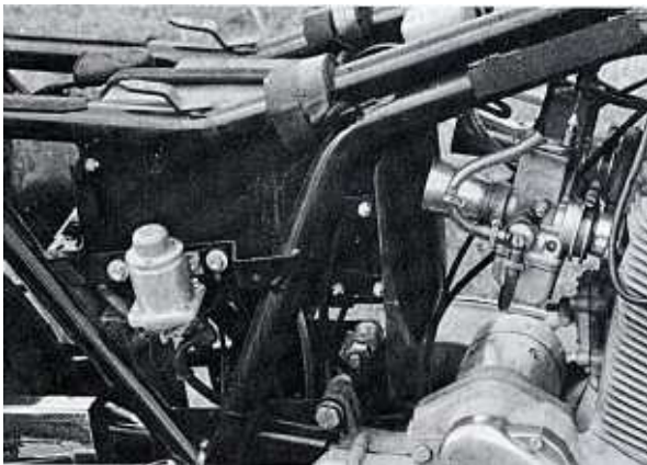
Bild 35 Der Batteriedeckel einer frühen Zweizylinder. An diesem Modell lässt sich der Deckel leicht abnehmen
