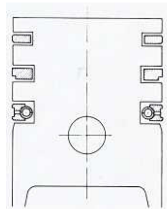
Bild 110 Schematischer Schnitt durch einen Kolben mit Kolbenringen für beide Modelle
