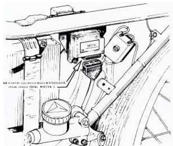
Bild 220 Der Elektronikkasten der BTZ an der SFC mit der Anleitung zum Auf-füllen des Steckers mit dem vorgeschriebenen Fett
