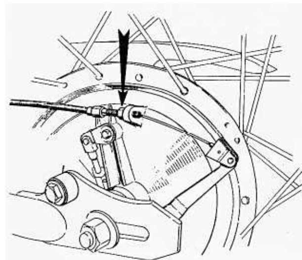
Bild 260 Die Laverda-Trommelbremse; der Pfeil zeigt auf die Gegenmutter der Einstellschraube
