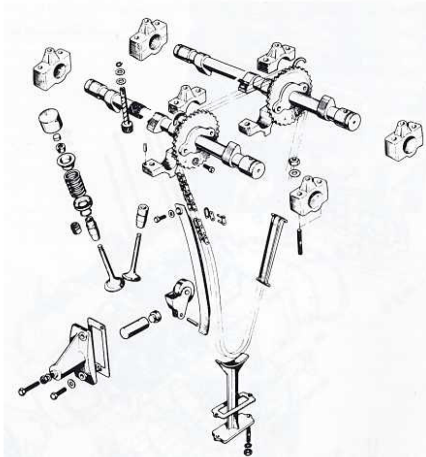
Bild 103 Die beiden obenliegenden Nockenwellen mit den Ventilen
