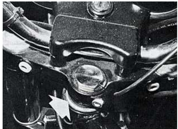
Bild 43 Das Lenkkopflager wird mit der schmalen Mutter unmittelbar unter der Gabelbrücke eingestellt
