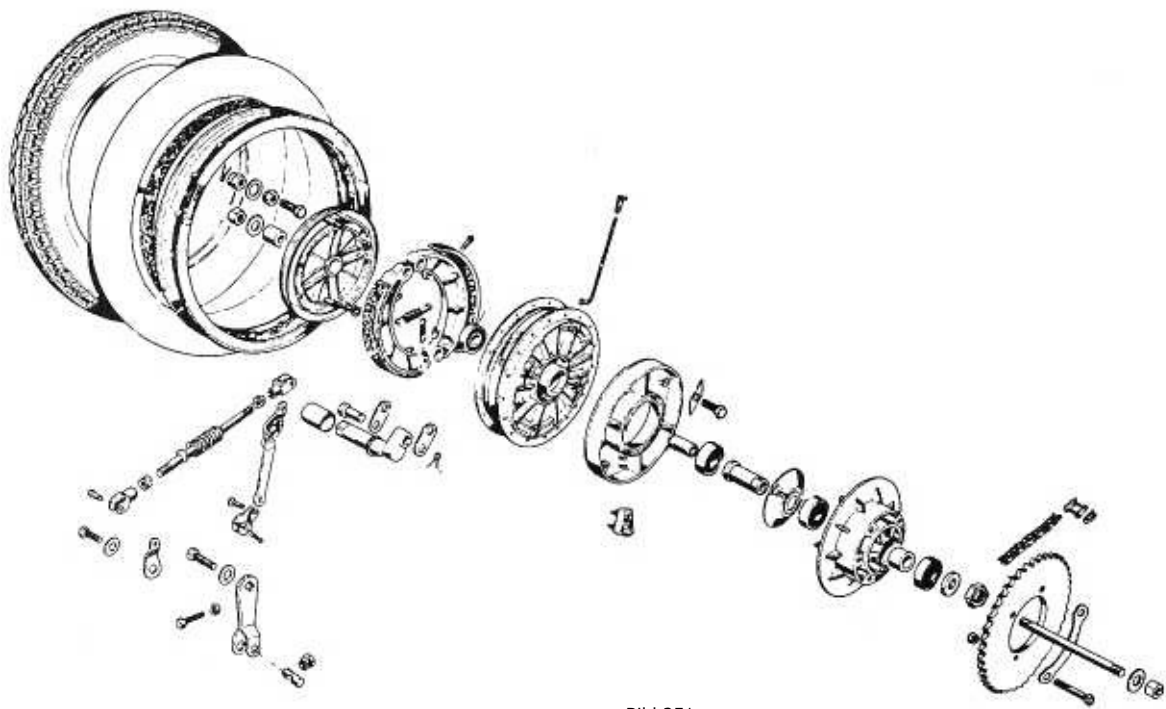
Bild 251 Die Laverda-Hinterradbremse
