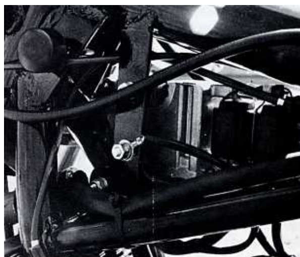
Bild 206 Das Steuergerät der HKZ von der anderen Seite. Am Rahmen eine Masseverbindung
