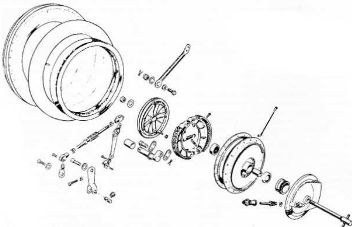
Bild 248 Die Laverda-Vorderradbremse
