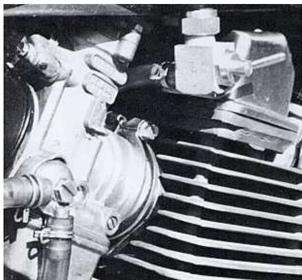
Bild 53 Diese Nahaufnahme des Benzinhahns zeigt recht gut, wie der Hahn zu zerlegen ist
