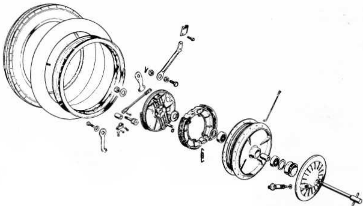
Bild 247 Die Grimeca-Vorderradbremse
