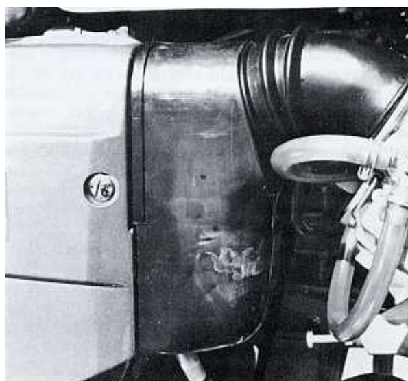
Bild 52 Der Filter der Dreizylinder sitzt hinter diesem schwarzen Deckel und der mit einer Schraube befestigten Seitenverkleidung
