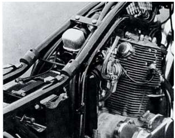
Bild 195 Der Lichtmaschinenregler zwischen den beiden oberen Rahmenrohren muss auf Gummi gelagert sein
