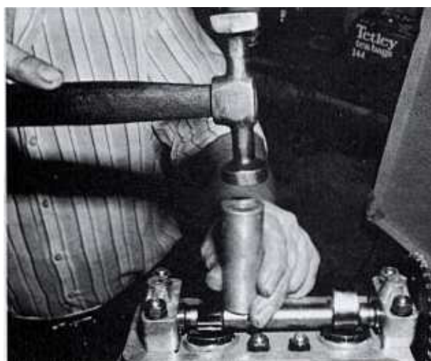
Bild 69 Vor dem endgültigen Anziehen der Nockenwellenlager klopft man mit einem weichen Dorn leicht auf die Welle, um sie in den Lagern zu zentrieren. Die Welle soll sich leicht drehen lassen
