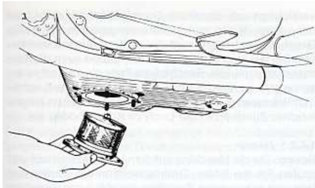
Bild 39 An den Zweizylindern dient der Ölfilterhalter auch als Ablassstopfen
