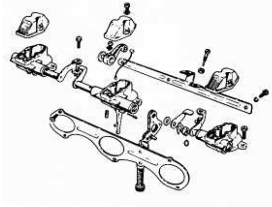
Bild 172 Die Anordnung der Dreivergaseranlage
