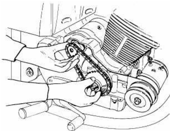
Bild 200 Einbau der endlosen Anlasserkette
