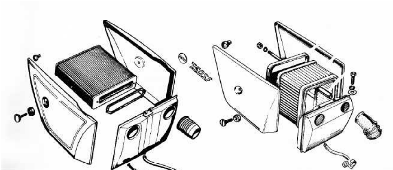
Bild 159 Der Luftfilter der ältesten Zweizylinder
