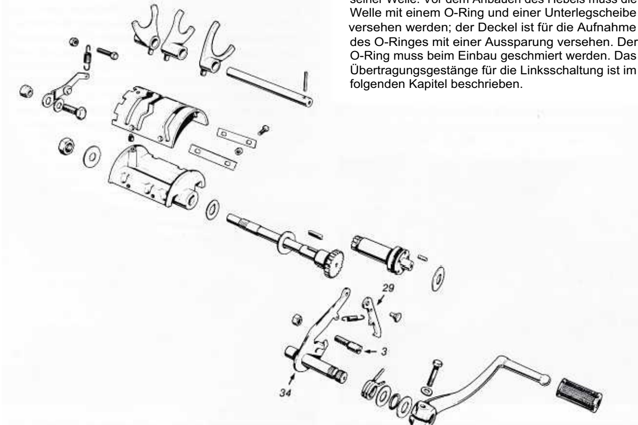
Bild 141 Der Schaltmechanismus der Zweizylindermaschine. Die Teile 29 und
