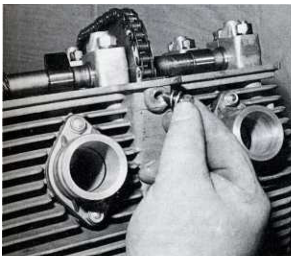
Bild 98 Die Befestigungsschraube der Gleitschiene des Kettenspanners
