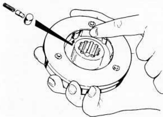
Bild 210 Die Einzelteile des Freilaufs an beiden Modellen. Alle Teile müssen gut geschmiert werden
