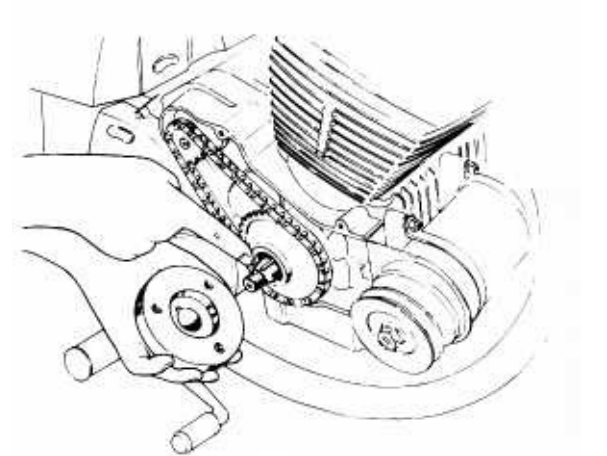
Bild 201 Die Nut im Anlasserfreilauf muss auf den Keil ausgerichtet werden
