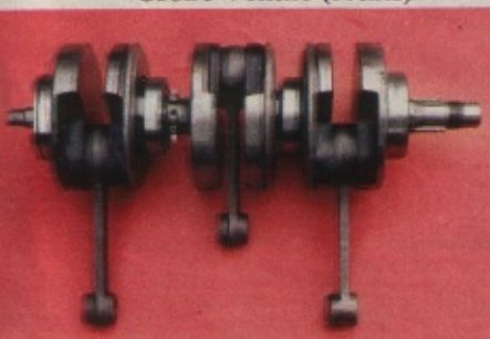
Serien-Kurbelwelle
